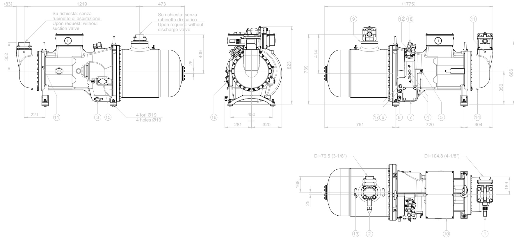
Fig. 49: dimensioni RS3-860-270 (MSI080 r.00);
